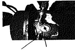
Stop en el cuerpo del acelerador Posición de potencia máxima
